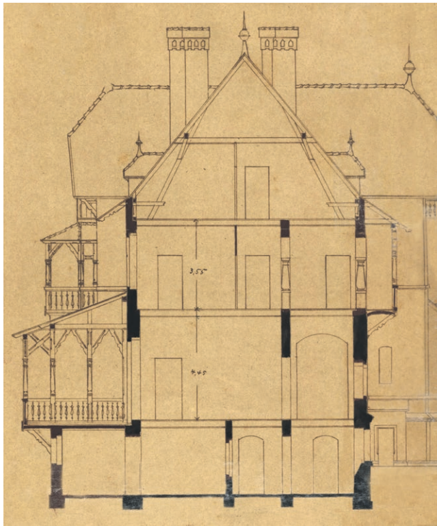
rysunek techniczny z 1894 roku
